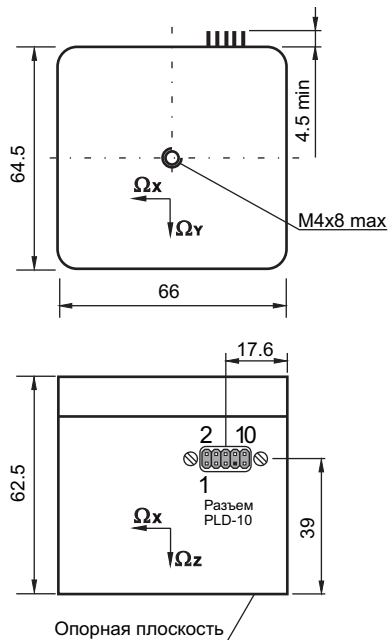
ГАБАРИТНО - УСТАНОВОЧНЫЙ ЧЕРТЕЖ
